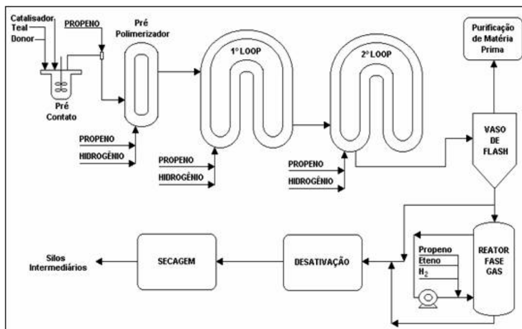
FIGURA x – Diagrama de processo Bulk1, Bulk2 e Piloto.
